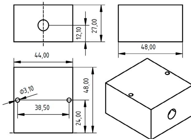
ASC 281 (Uniaxial)
