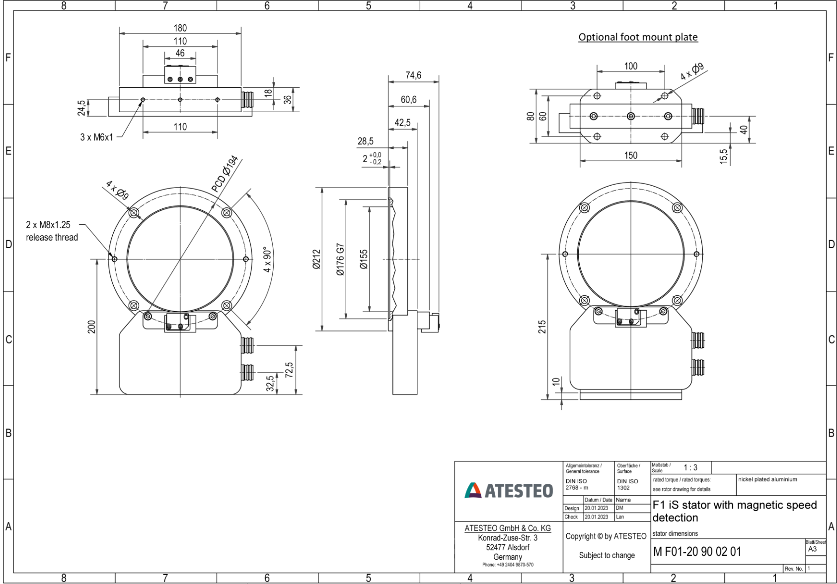
F1iS - Stator - speed magnétique
