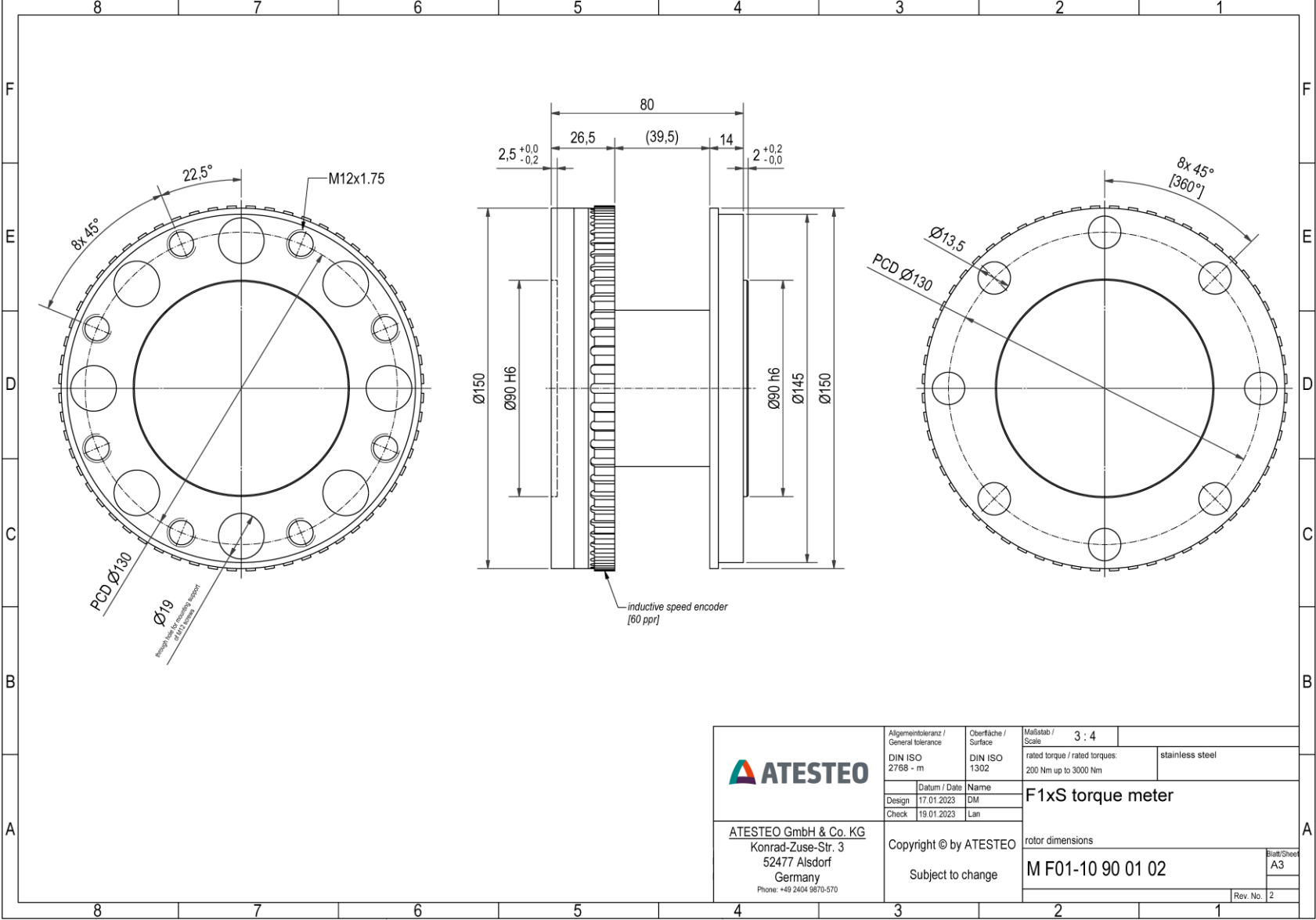
F1iS - Rotor - no speed
