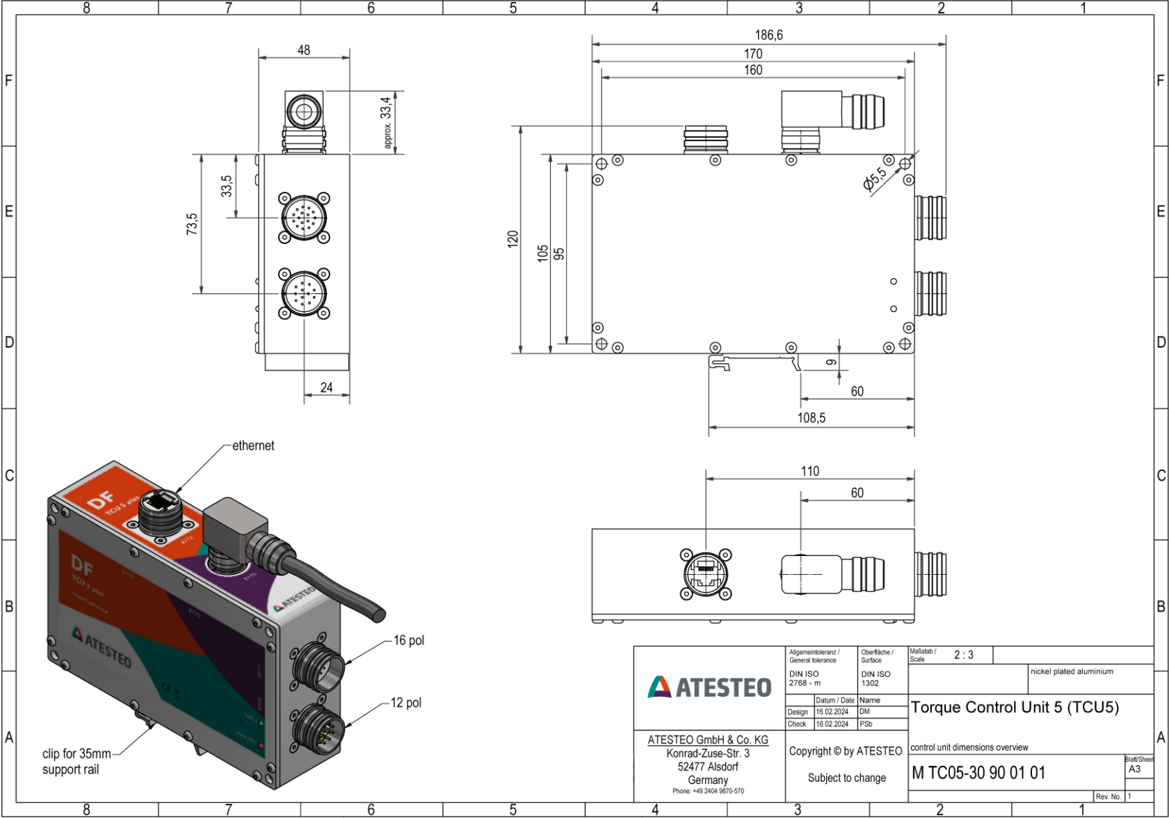
DF4 dual - TCU
