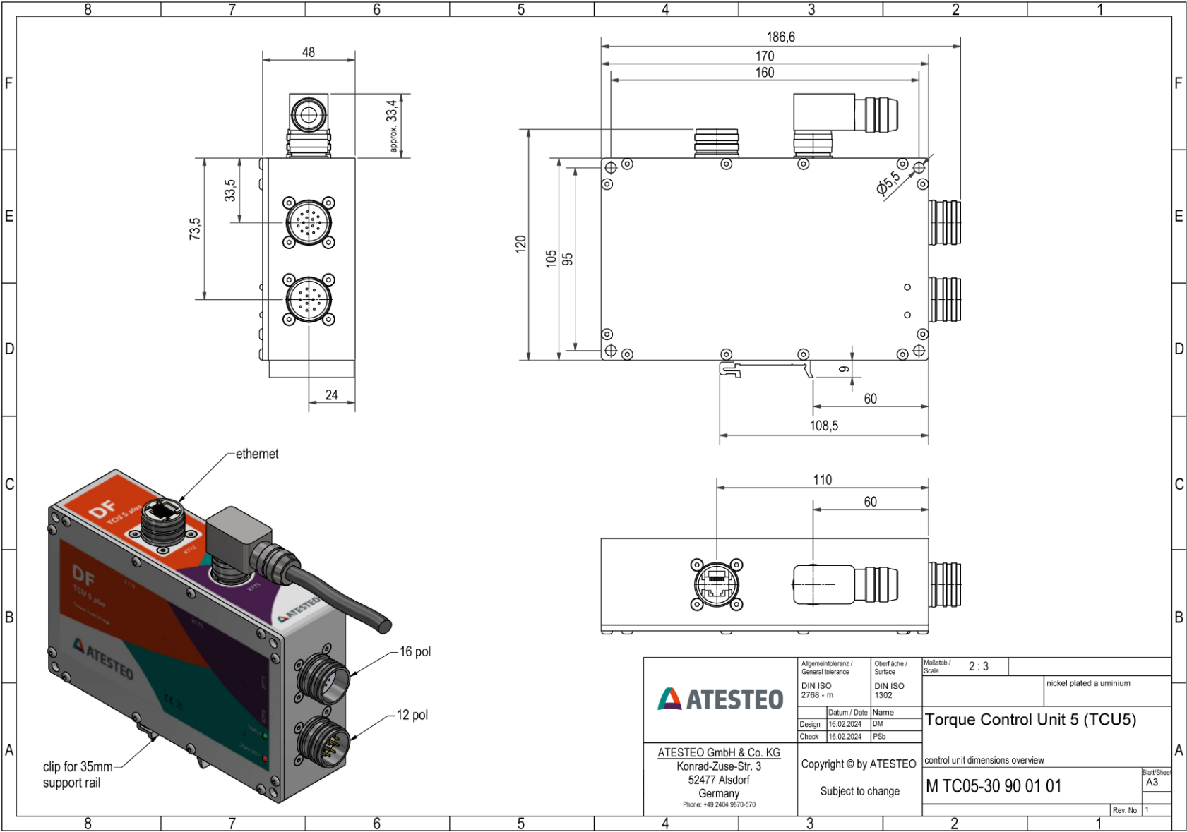
DF3 dual - TCU
