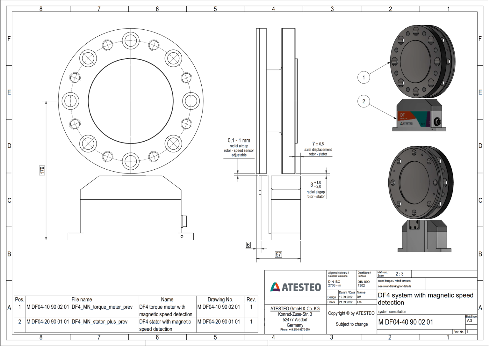
Ensemble rotor / stator - DF4 plus - avec sortie vitesse
