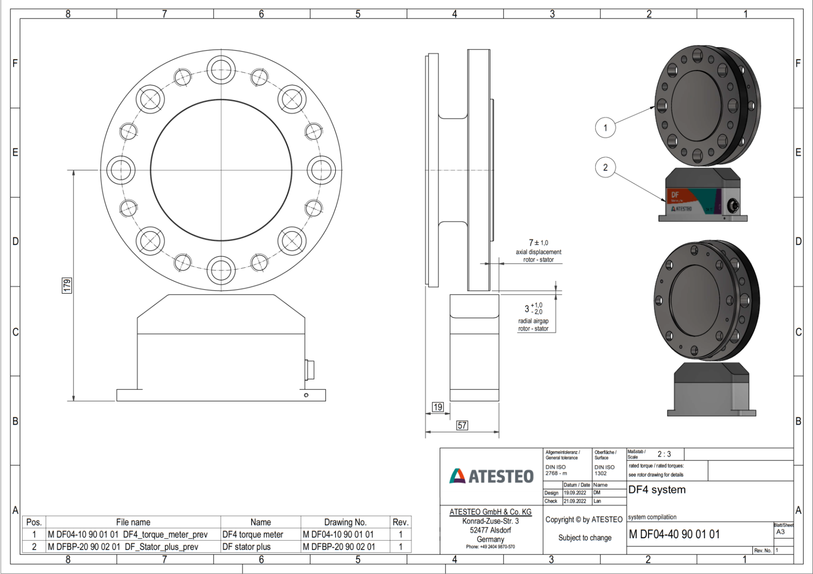
Ensemble rotor stator - DF4 plus - sans sortie vitesse
