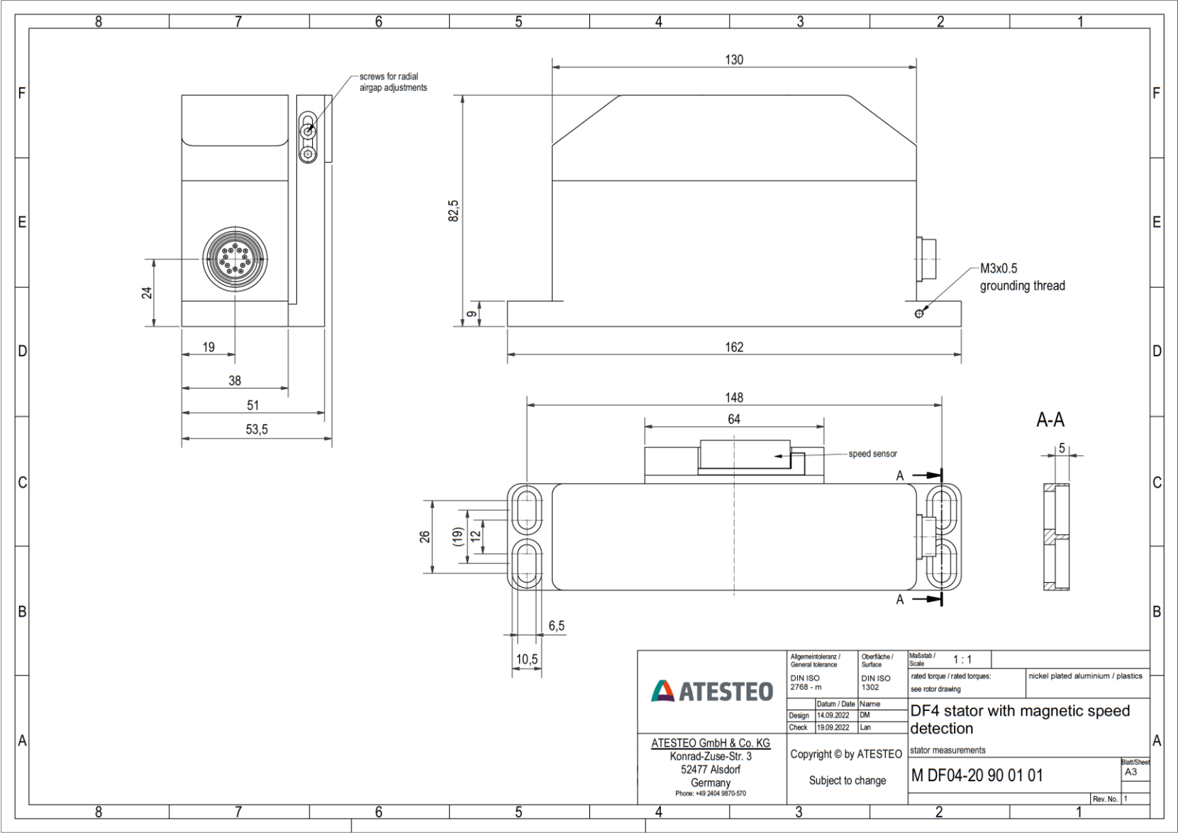
Plan stator - DF4 plus - avec sortie vitesse
