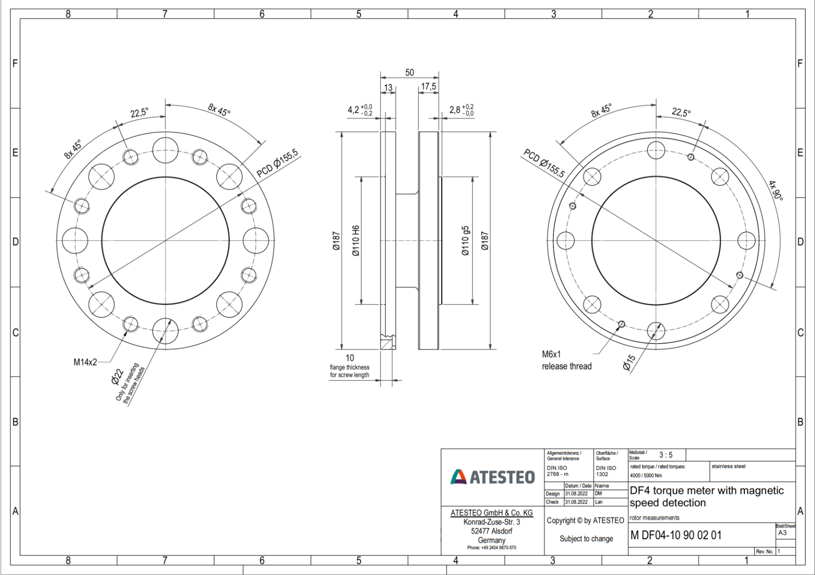
Plan rotor - DF4 plus - avec sortie vitesse
