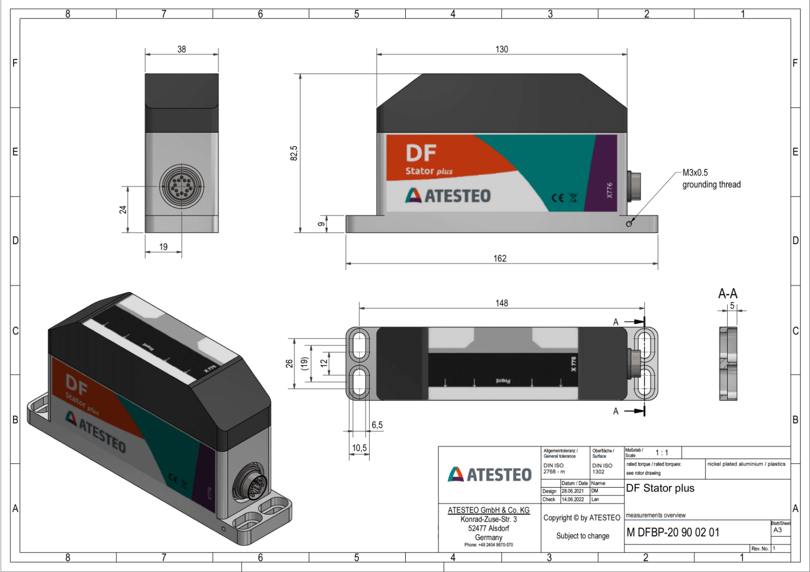
Plan stator - DF4 plus - sans sortie vitesse
