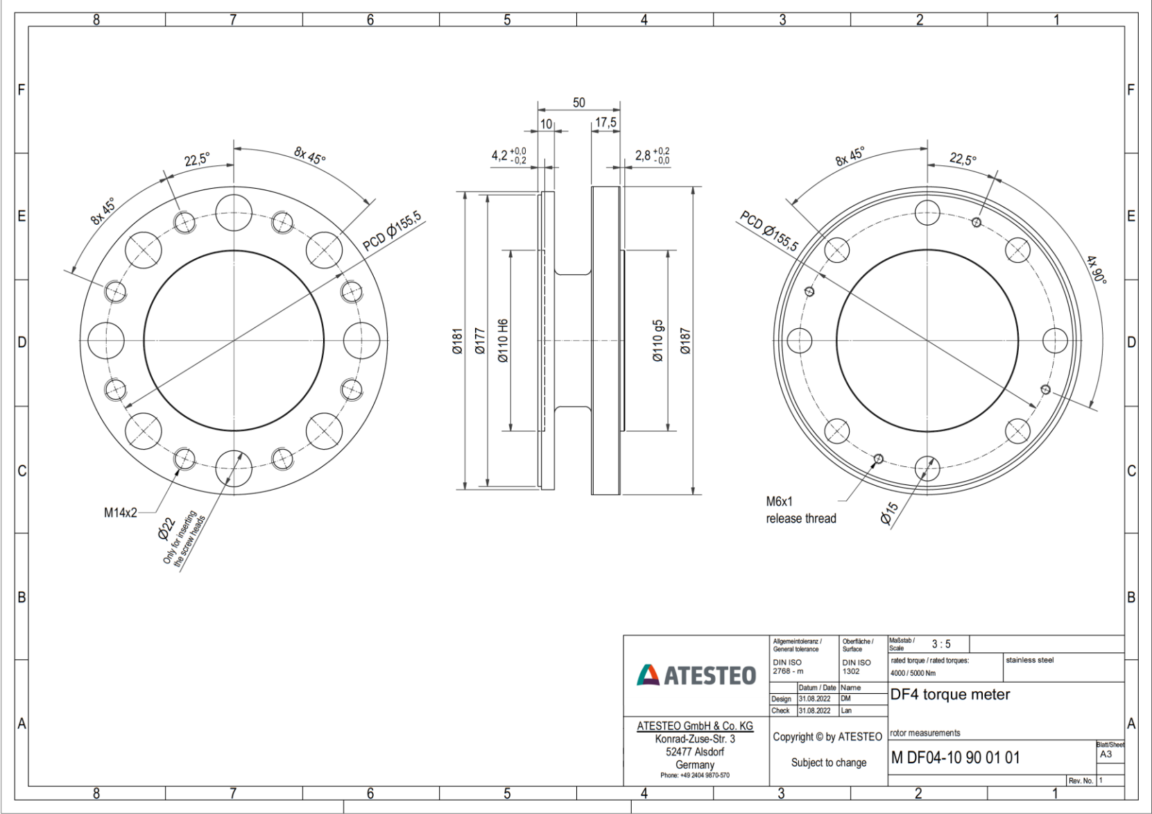
Plan rotor - DF4 plus - sans sortie vitesse
